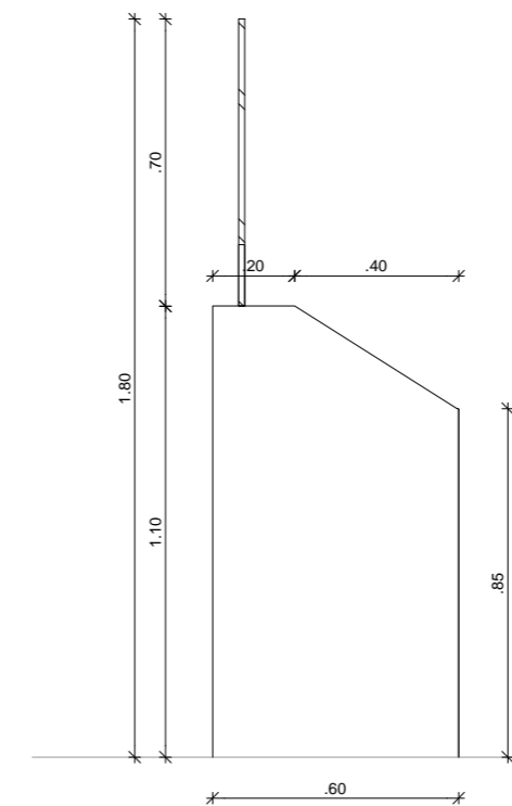
STRANSKI POGLED
