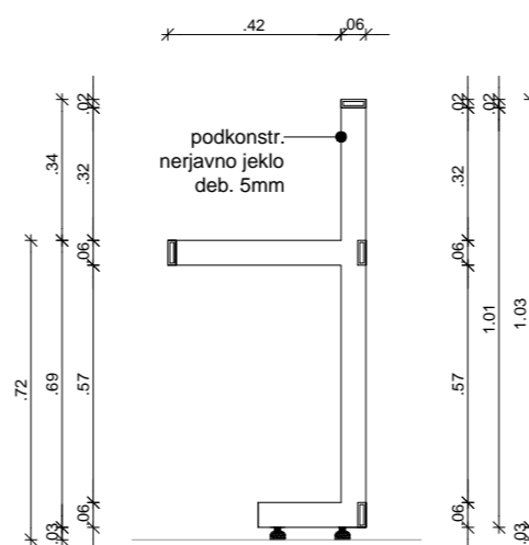
SREDINSKA PODKONSTRUKCIJA
