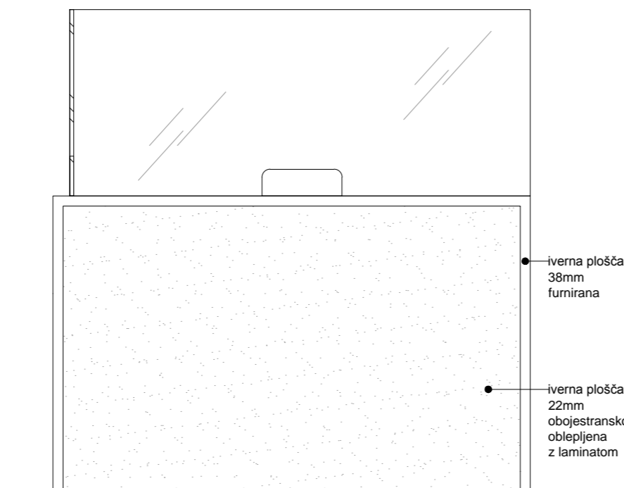
POGLED
