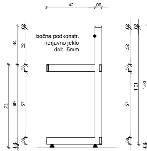
BOČNA PODKONSTRUKCIJA
