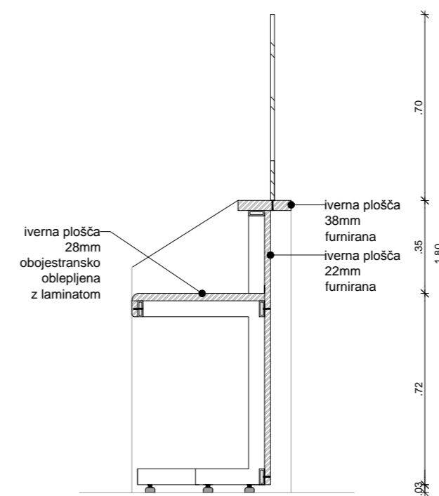
STRANSKI POGLED
