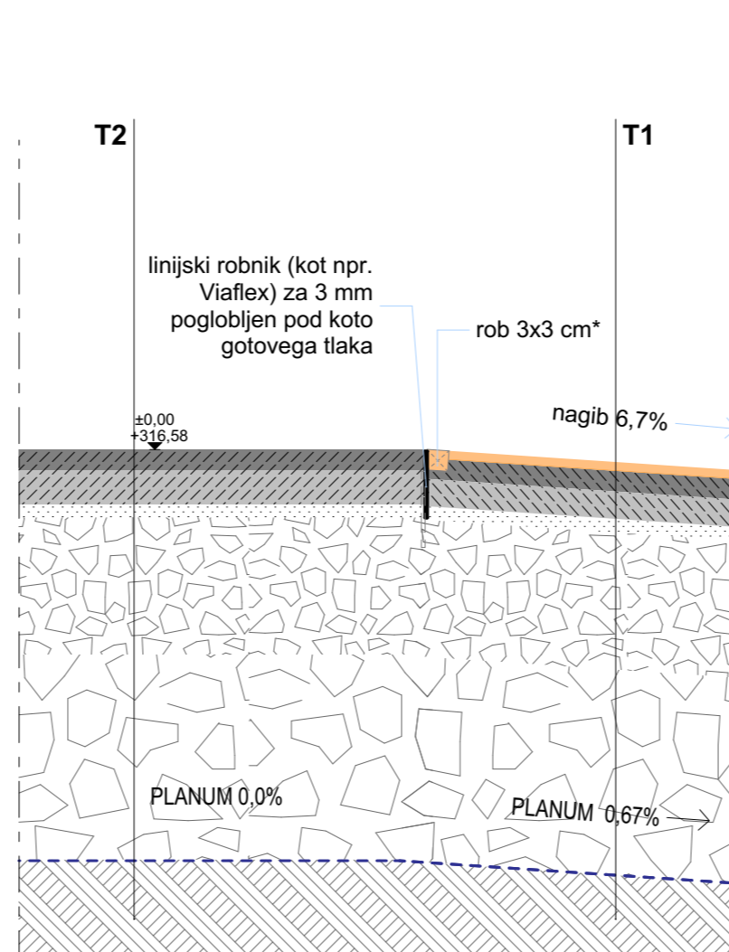
S4 - stik med sintetično športno podlago in asfaltom
