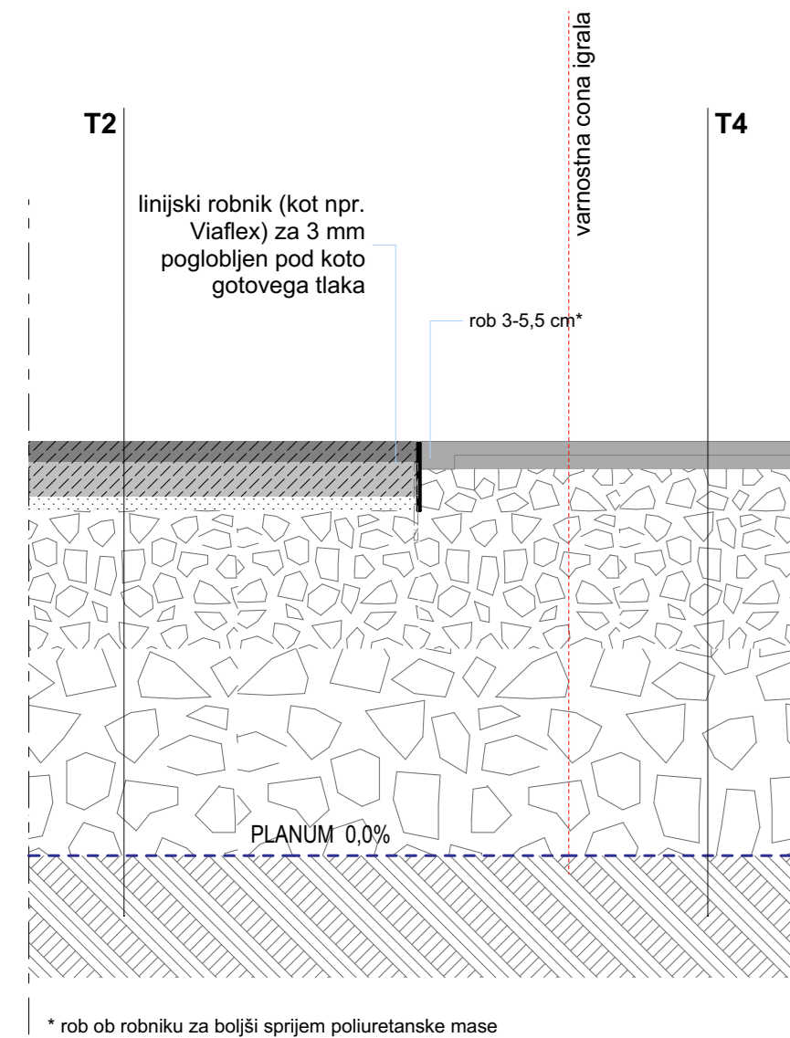
S1 - stik med asfaltom in sintetično varnostno podlago
