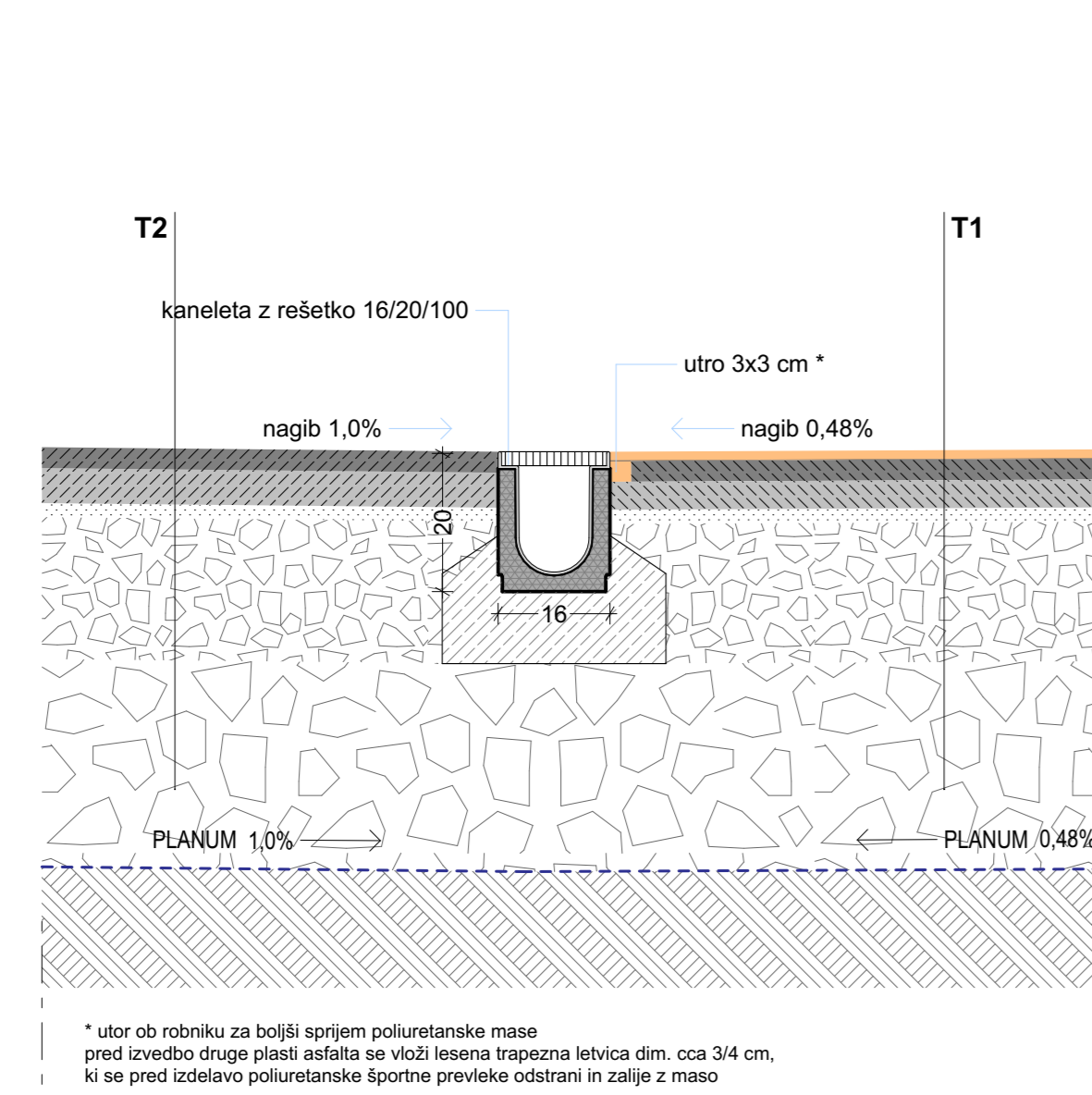
S2 - stik med asfaltom, kaneleto in sintetično športno podlago
