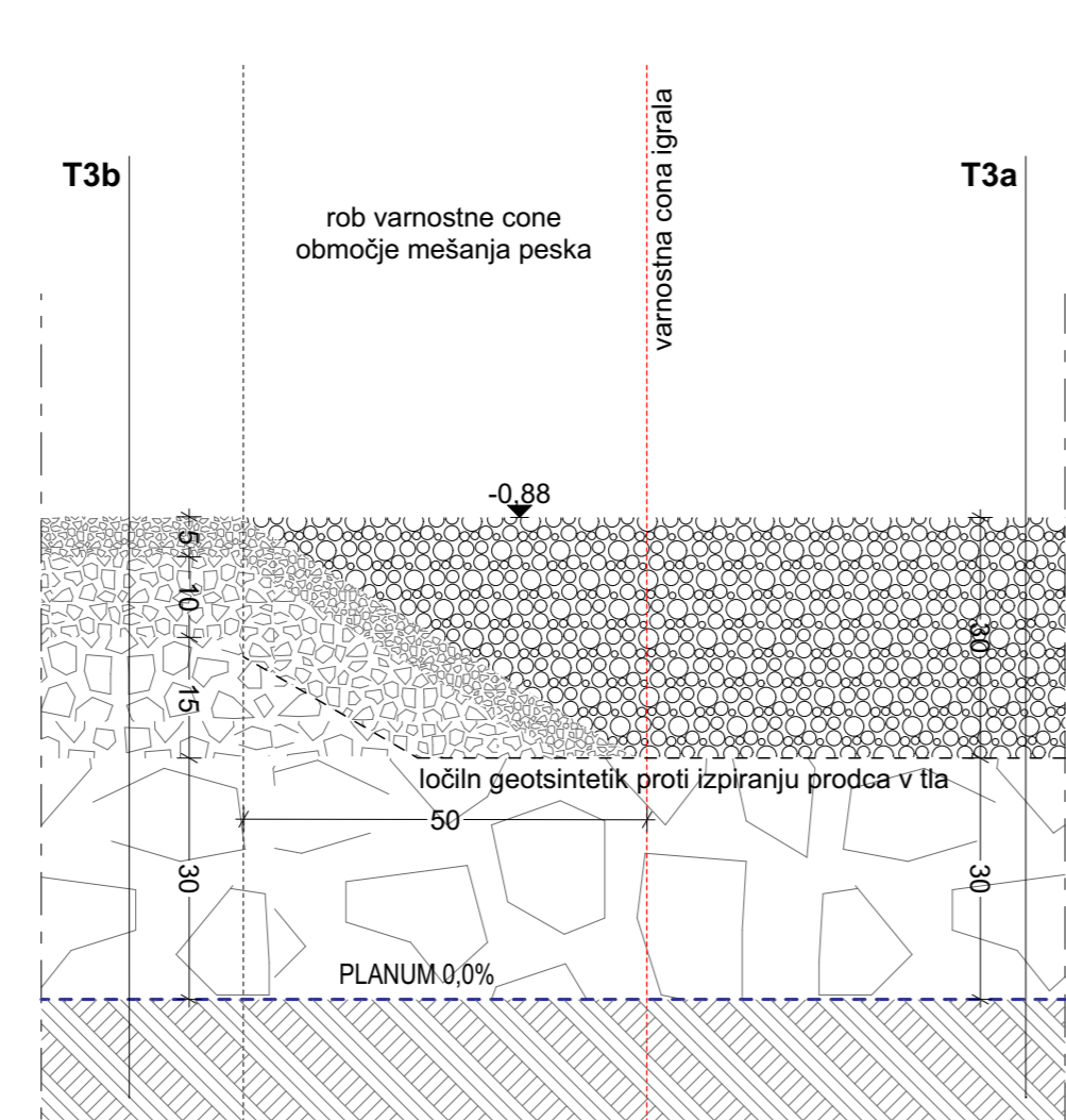
S3 - stik med drobljencem in prodcem
