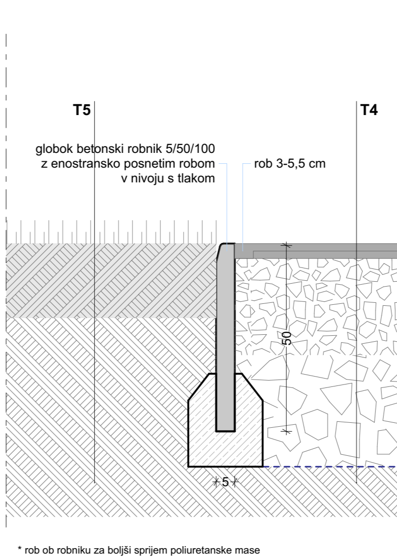
S6 - stik med travo in varnostno podlago
