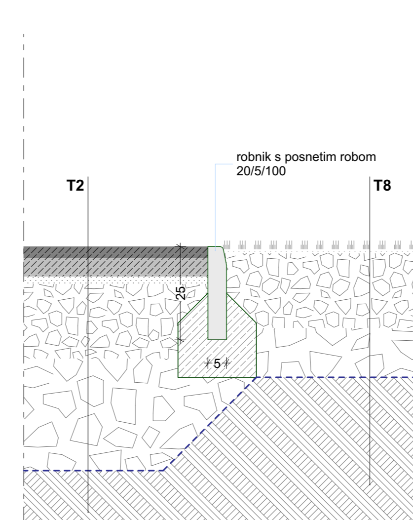
S5 - stik med asfaltom in umetno travo
