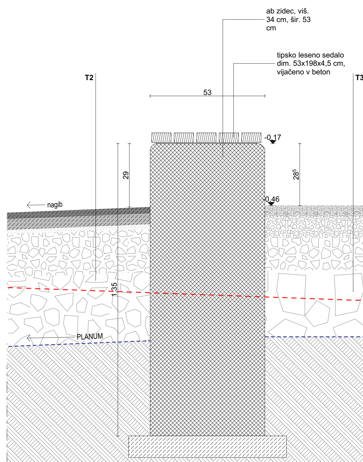
S7 - stik med asfaltom, klopjo in drobljencem
