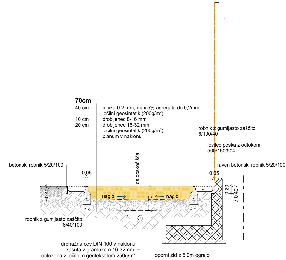
prečni prerez A-A
